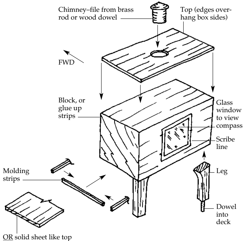
FIG. 32 - Binnacle
